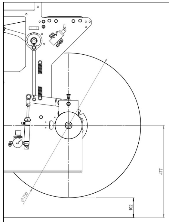
Fig. 2 - Bobina
