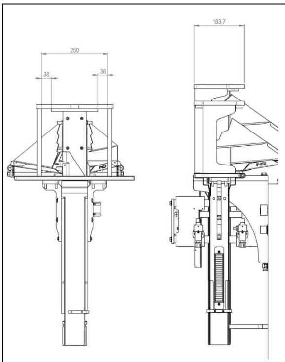
Fig. 1 - Tubo formatore
