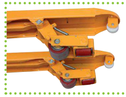
▶ Particolare rulli LT4V con traslazione frontale e laterale
